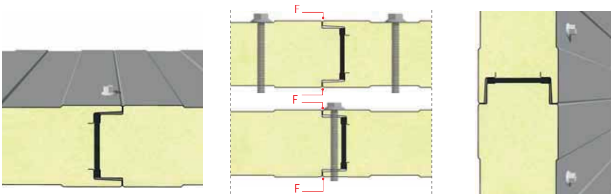
Modalità di fissaggio dei pannelli
